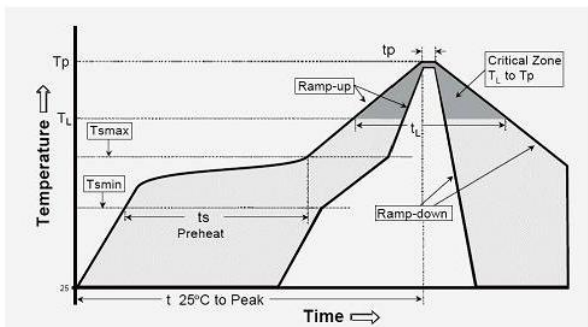
附录 4：炉温曲线图
